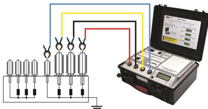
Conexión del DEM60R al transformador trifásico
